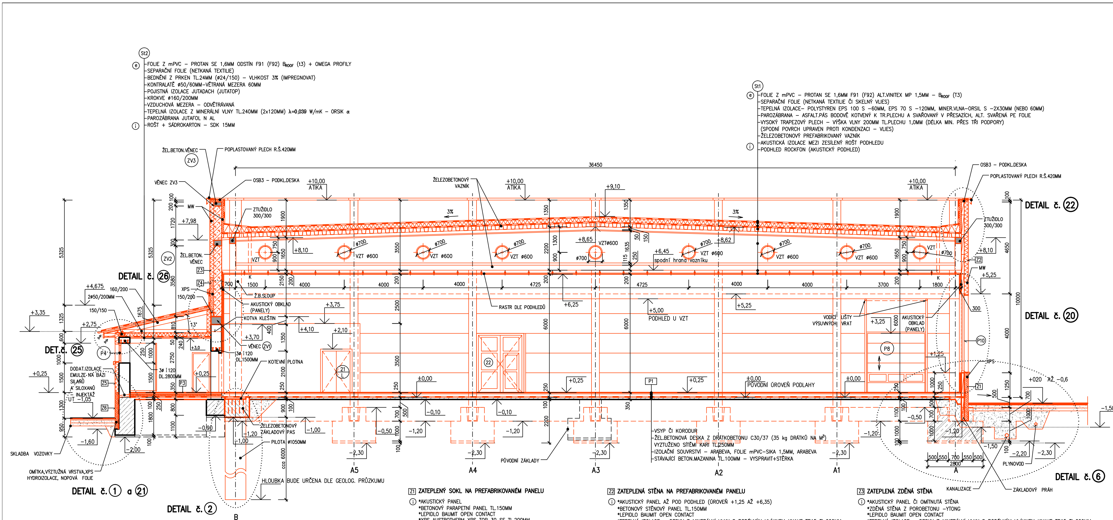
PŘÍČNÝ ŘEZ 1-1 1:100
