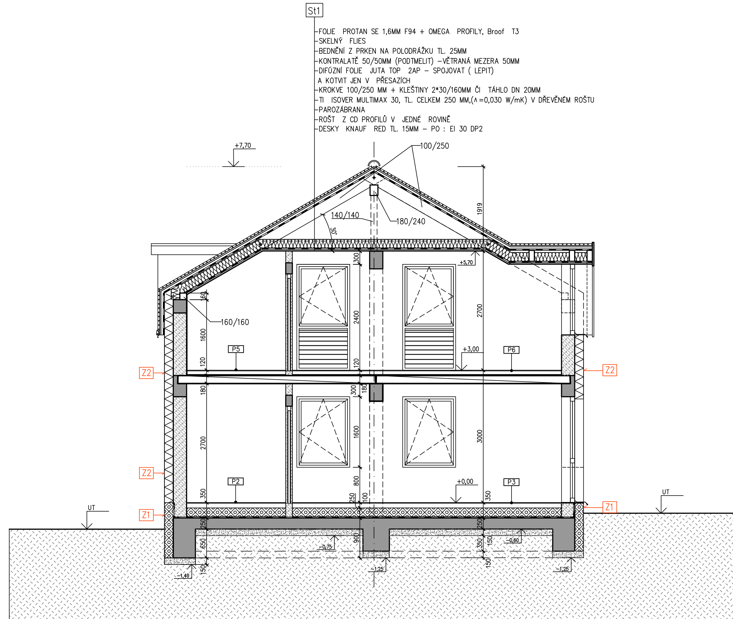
ŘEZ A-A 1:50
