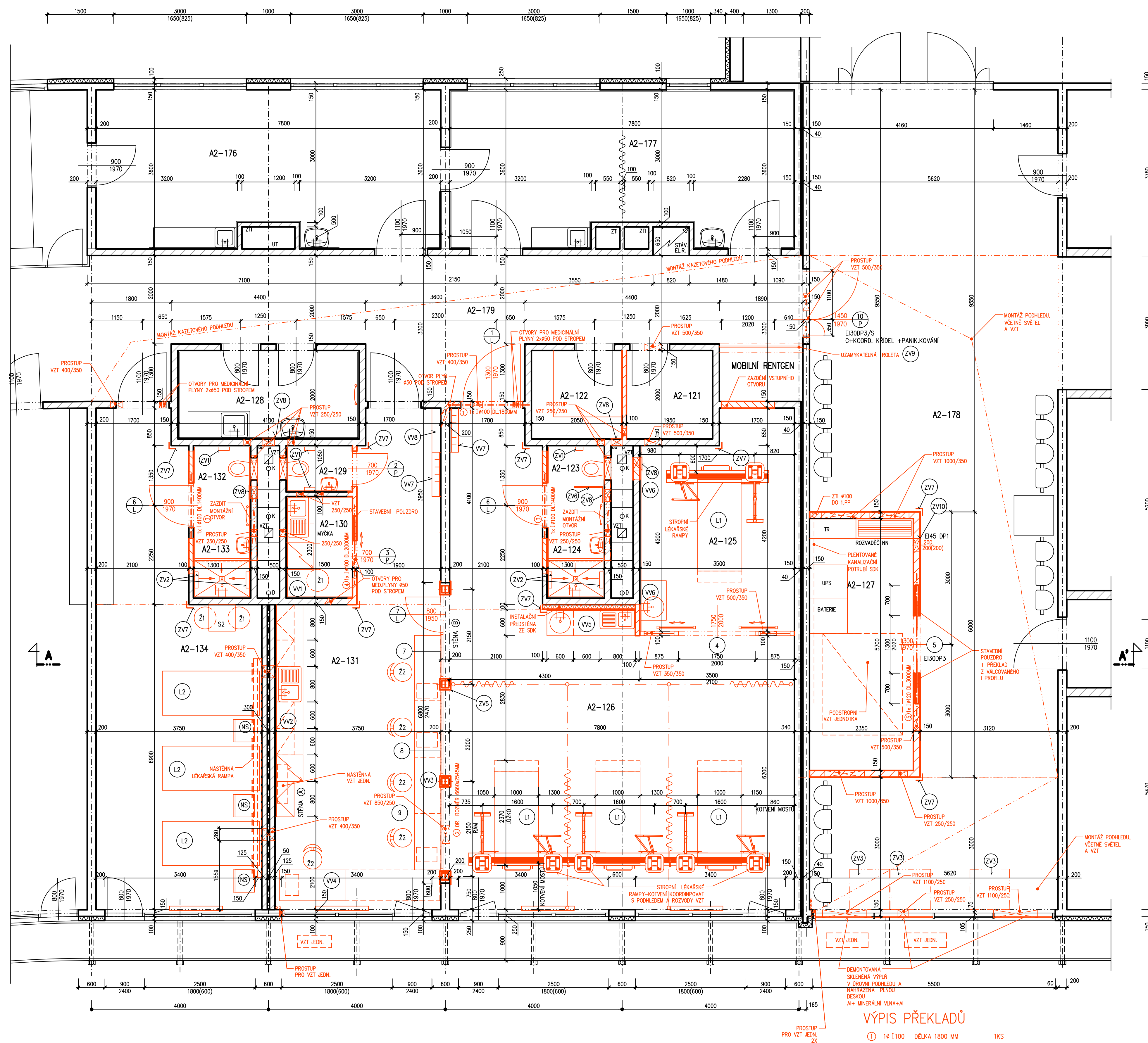
PŮDORYS 1.NP 1:50
