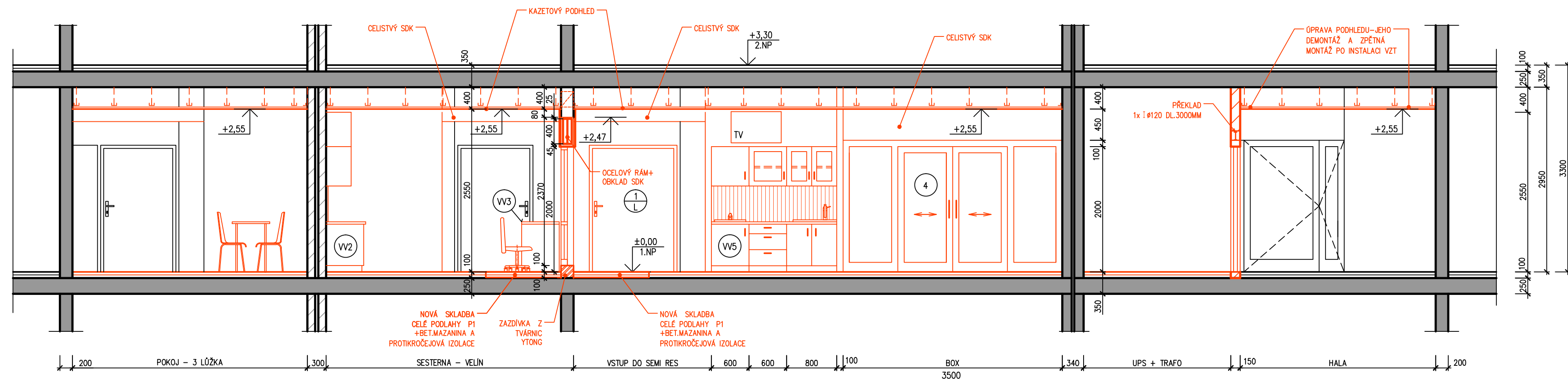
ŘEZ A-A' 1:50
