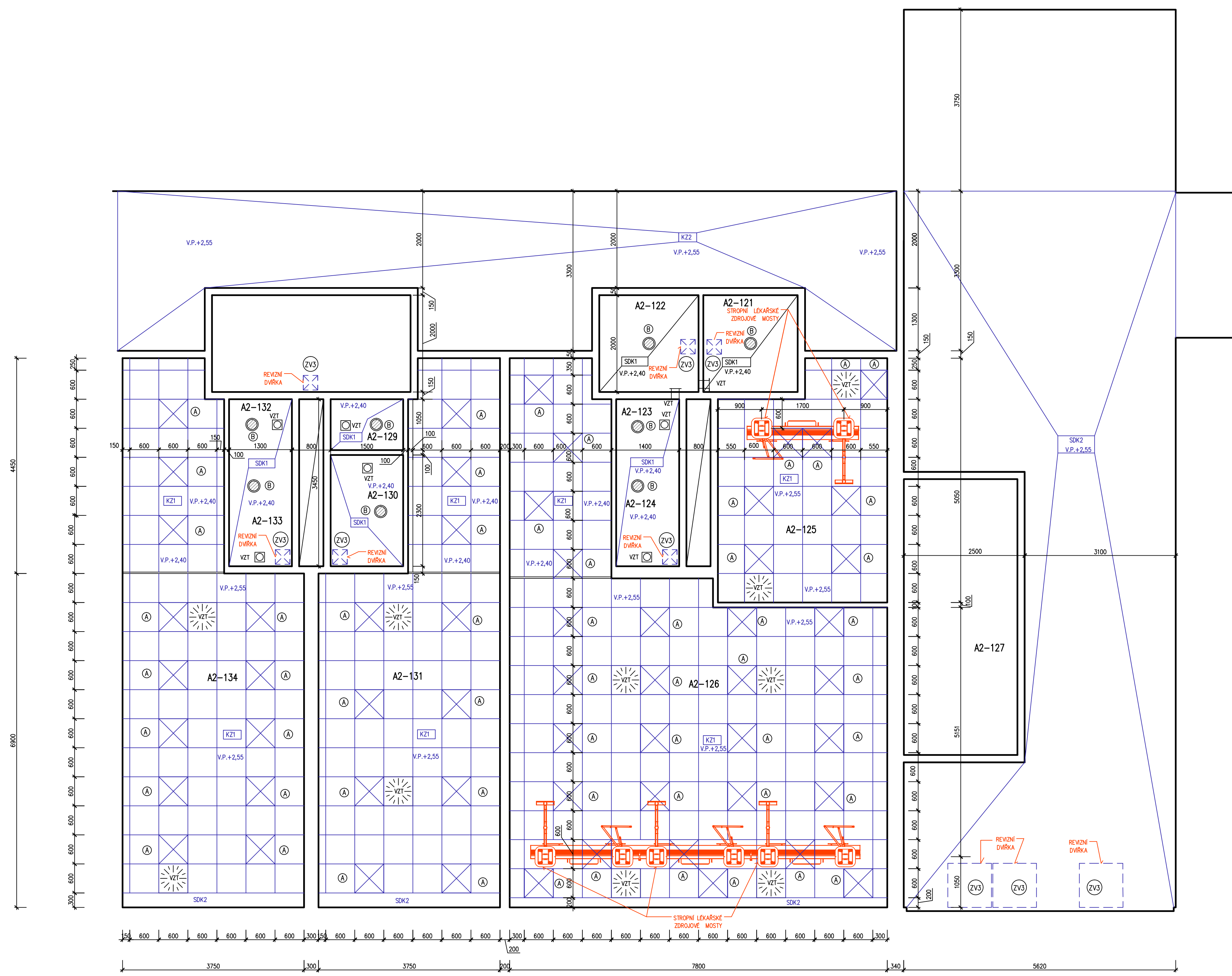
PODHLÉDY 1:50
