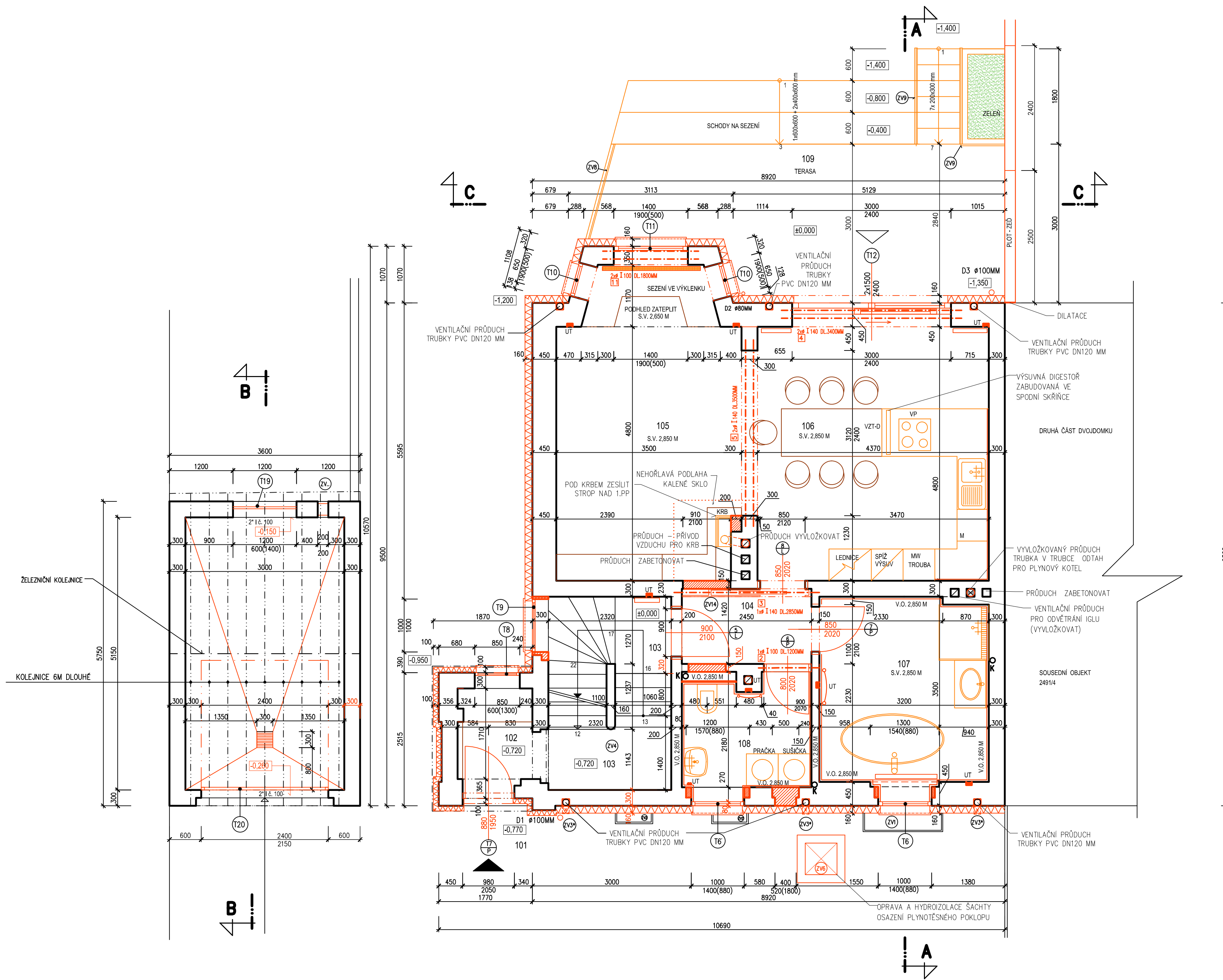
PŮDORYS 1.NP – NOVÝ STAV
