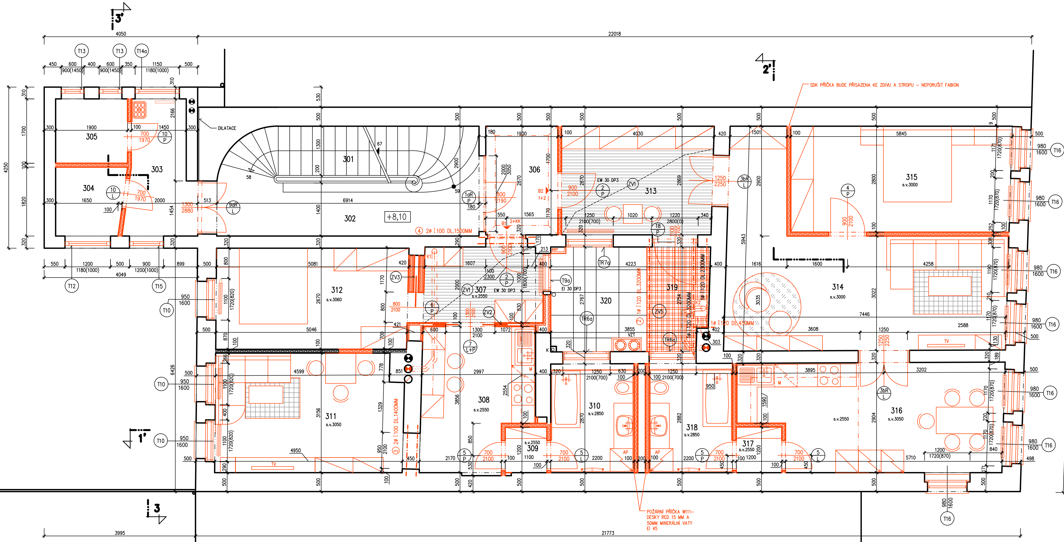
PŮDORYS 3.NP – NOVÝ STAV 1:50
