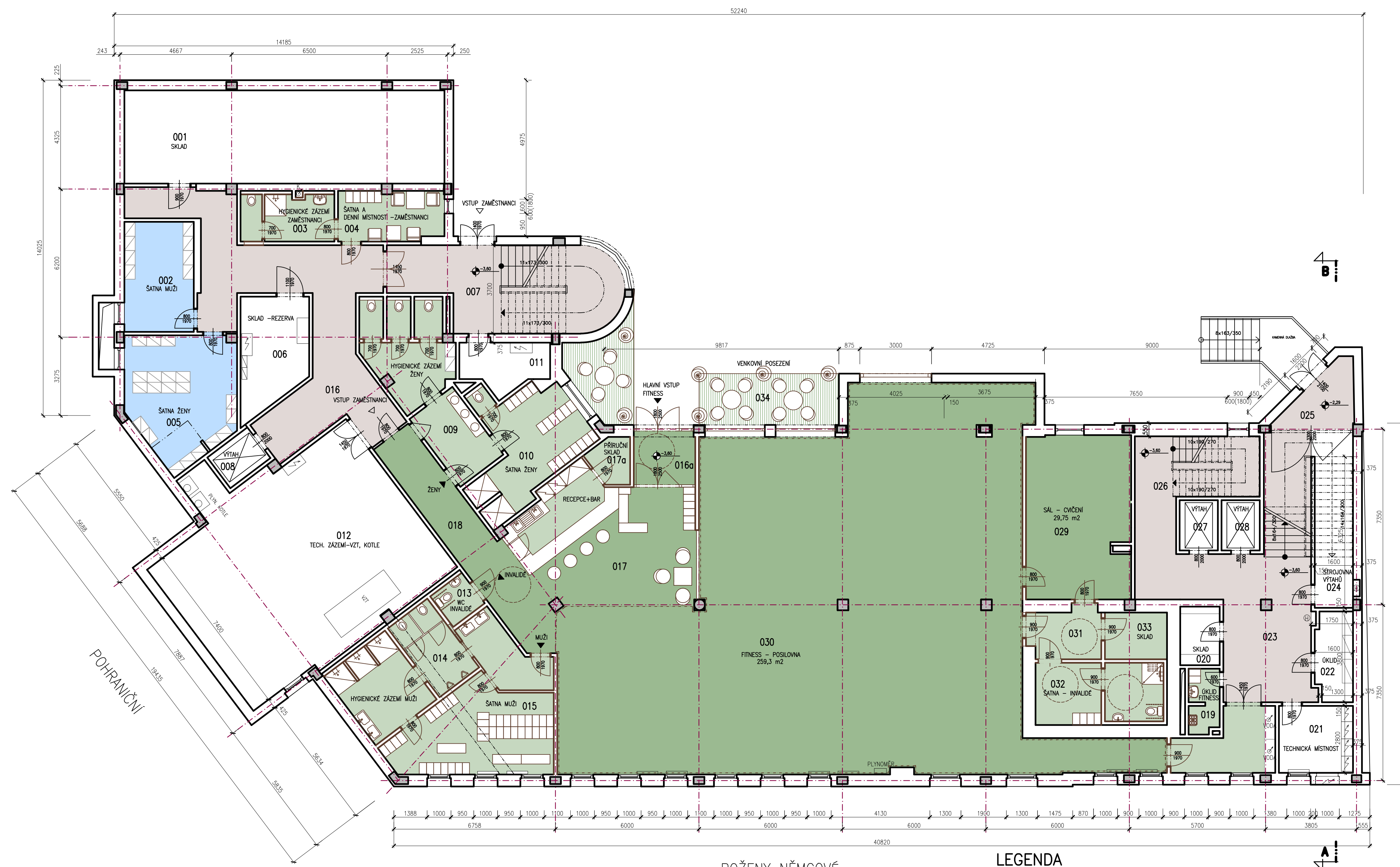
PŮDORYS 1.PP – NÁVRH –VARIANTA A M • 1:100 FITNESS
