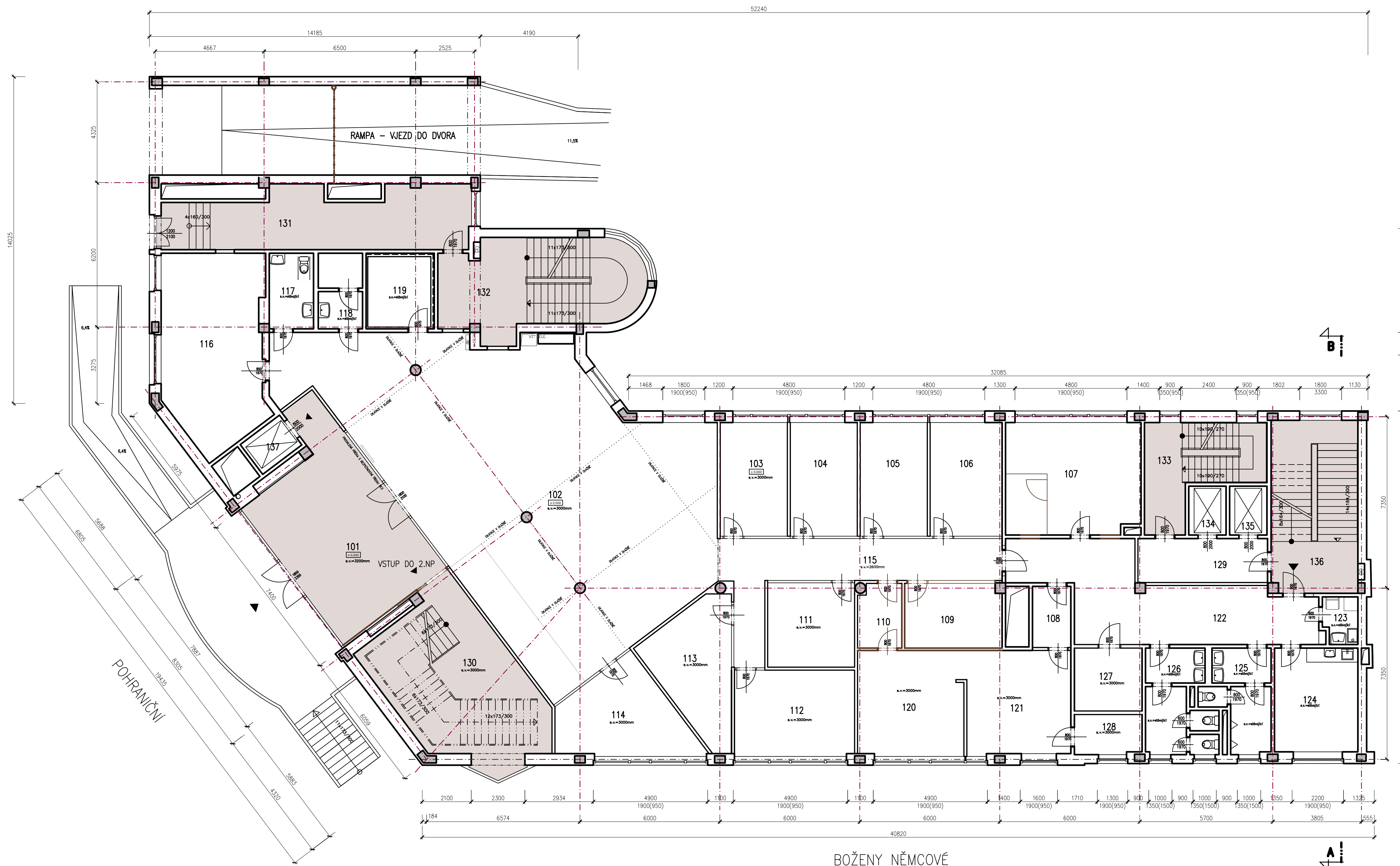
PŮDORYS 1.NP – NÁVRH – VARIANTA A M • 1:100
