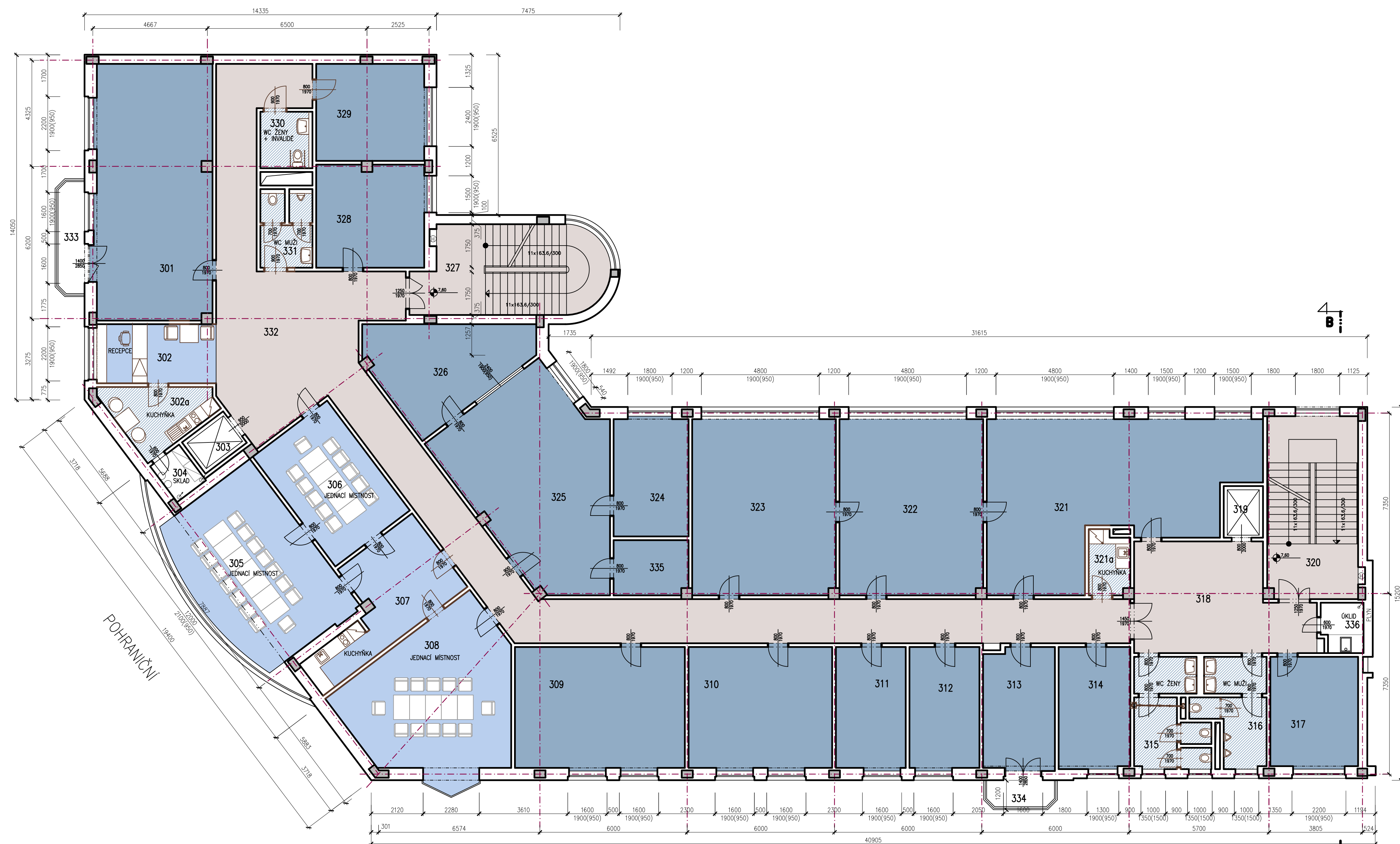
PŮDORYS 3.NP – NÁVRH – VARIANTA (A) M • 1:100 KANCELÁŘE
